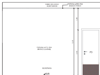
4 VISTA 3 ESCALA: 1 : 25
