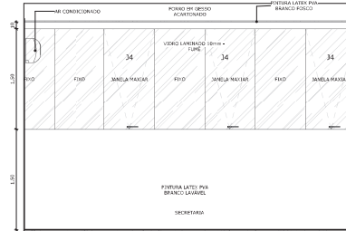
3 VISTA 2 ESCALA: 1 : 25
