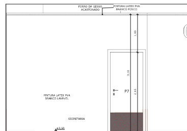
5 VISTA 4 ESCALA: 1 : 25
