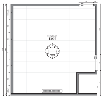
1 SECRETARIA ESCALA: 1 : 25
