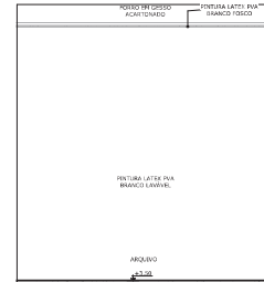
10 VISTA 8 ESCALA: 1 : 25
