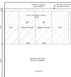
8 VISTA 6 ESCALA: 1 : 25
