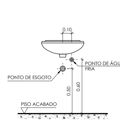
VISTA FRONTAL ESCALA 1:25 LAVATÓRIO
