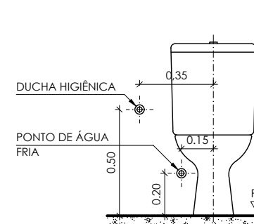
VISTA FRONTAL ESCALA 1:25 BACIA SANITÁRIA
