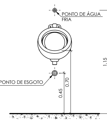
VISTA FRONTAL ESCALA 1:25 MICTÓRIO
