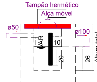
Caixa de gordura - FUNDAÇÃO Corte 1 - ESC. 1:25
