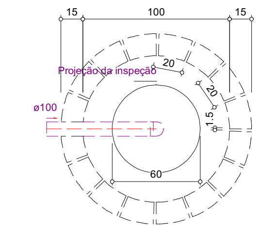
Sumidouro - FUNDAÇÃO Planta baixa - ESC. 1:25
